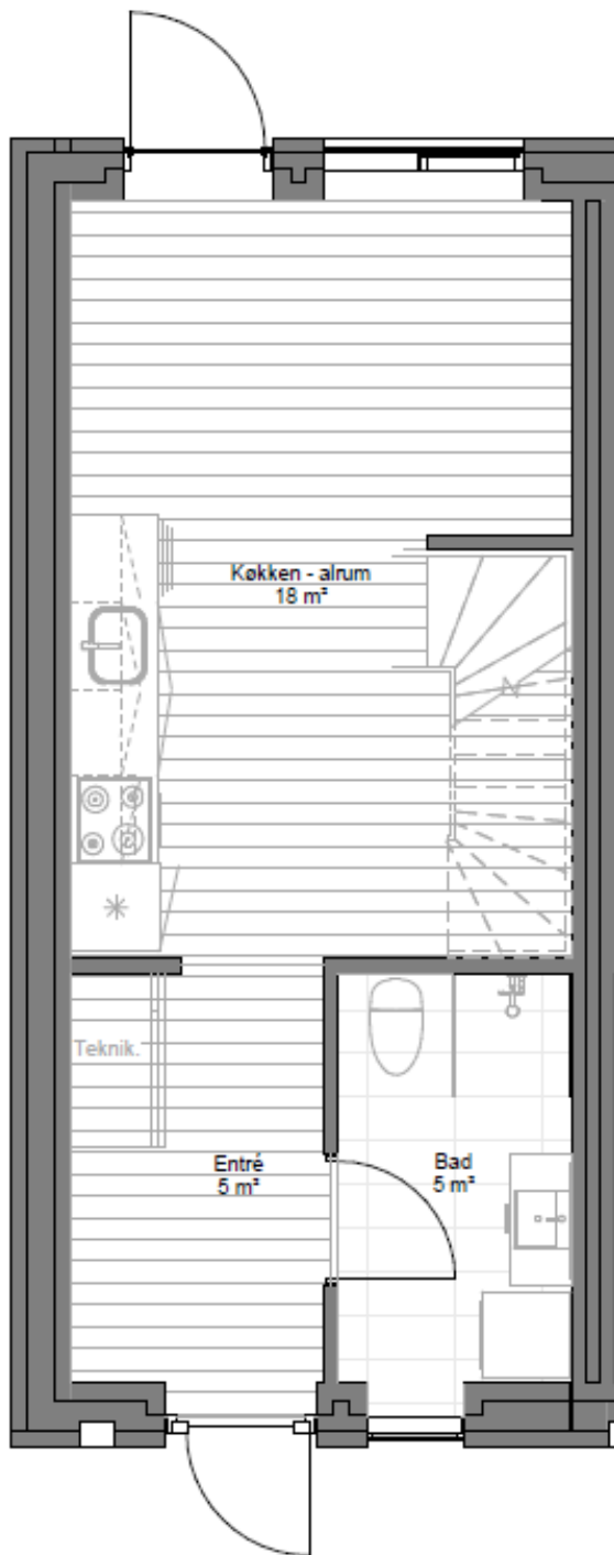
Stueplan
